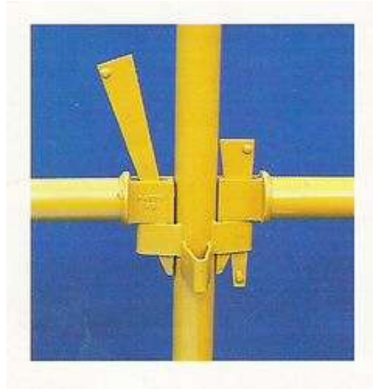
kwikstage system.jpg
